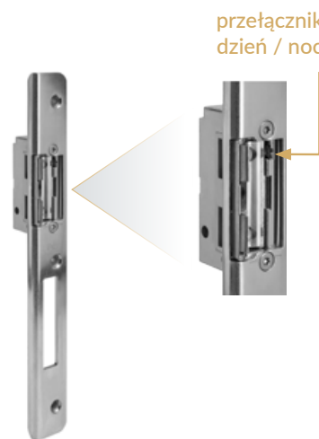
Elektrozaczep
