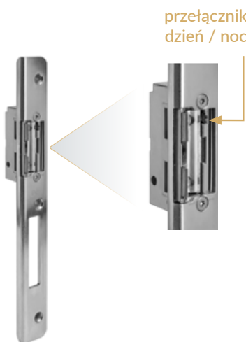
Zaczep współpracujący z antabą
