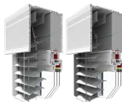
ŻALUZJA NAKŁADANA Z PROFILEM C80 / Z90
