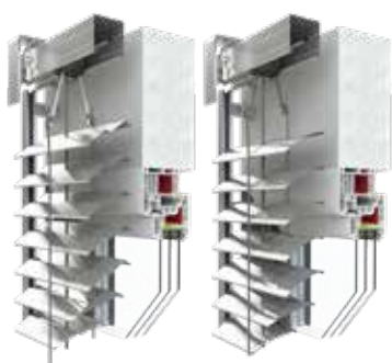
ŻALUZJA STANDARDOWA Z PROFILEM C80 / Z90
